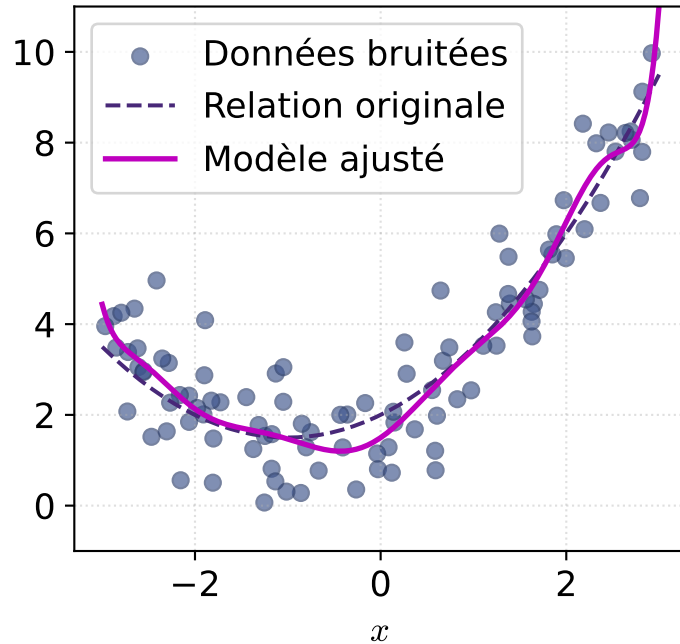
Sans régularisation
