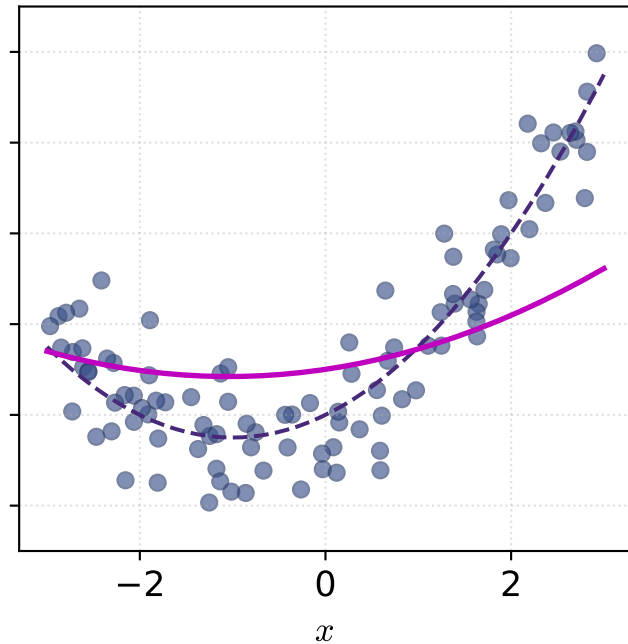
Lasso (alpha=1)
